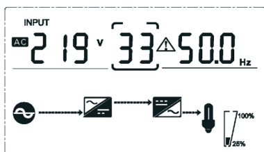
(2) Входные параметры
