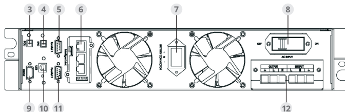
Вид сзади
