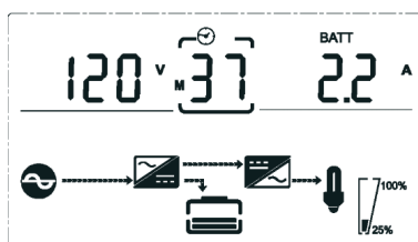
(5) Напряжение и ток АКБ- (отрицательной группы АКБ)
