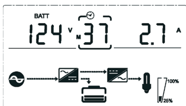
(4) Напряжение и ток АКБ+ (положительной группы АКБ)
