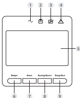
Общий вид пульта управления
