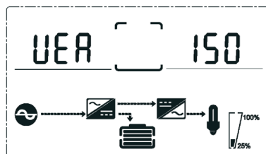
(9) Версия программного обеспечения
