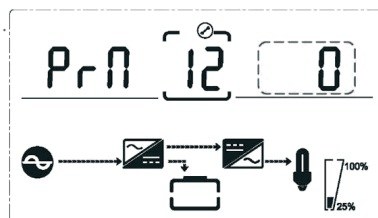
Настройка количества резервных модулей для параллельного режима (Примечание: часть изображения, выделенная пунктиром, мигает).
