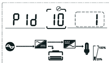
Настройка идентификатора для параллельного режима (Примечание: часть изображения, выделенная пунктиром, мигает).
