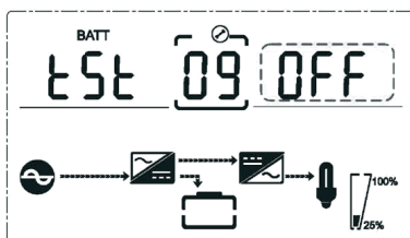
Настройка тестирования АКБ
