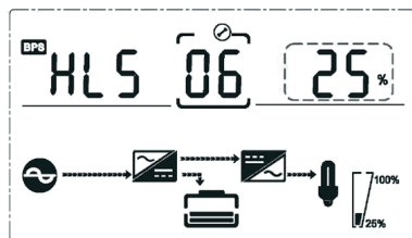
Настройка максимального напряжения байпаса
