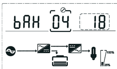
Настройка емкости АКБ
