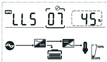
Настройка минимального напряжения байпаса
