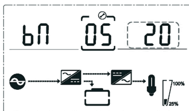
Настройка количества АКБ
